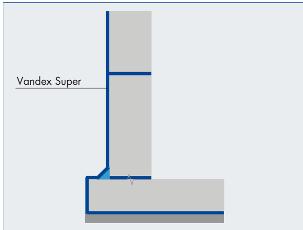
Pamatų hidroizoliavimas iš išorės
