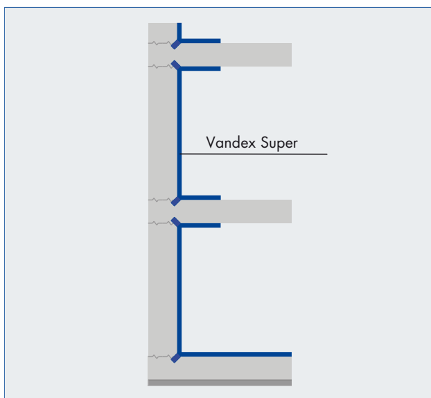
Daugiaaukščio parkingo hidroizoliavimas
