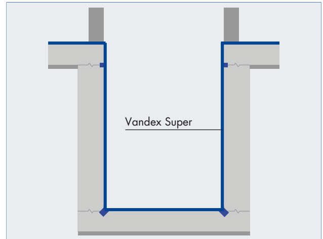
Lifto šachtos hidroizoliavimas iš vidaus
