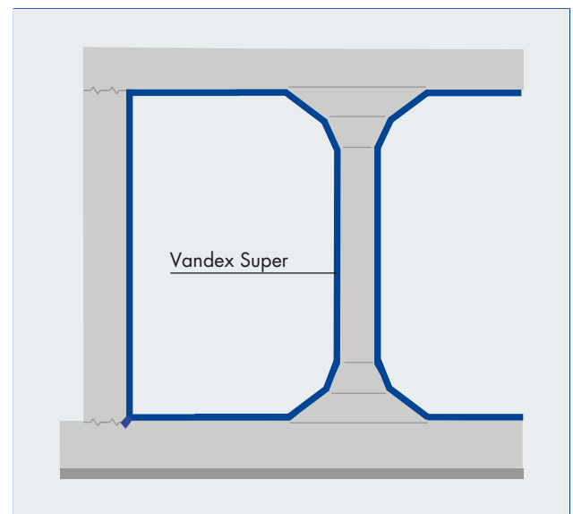
Geriamo vandens rezervuaro hidroizoliavimas
